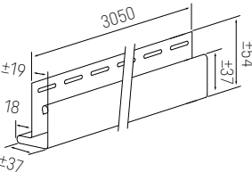
SV(P) 12.5 Outside corner mini
